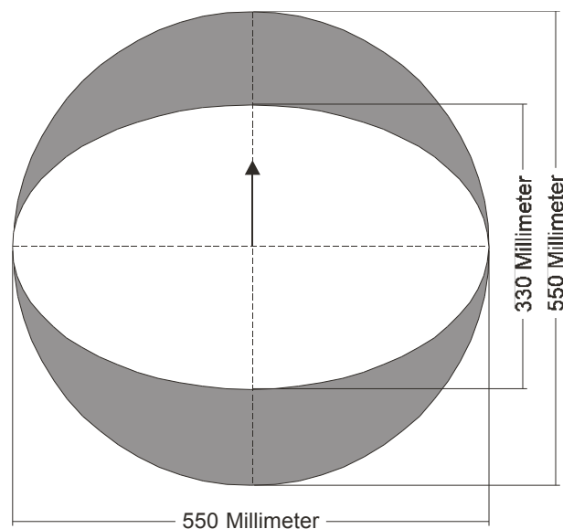
Bild 1 Aufsicht auf Zigarettenträger mit Überlappungsflächen (grau)
